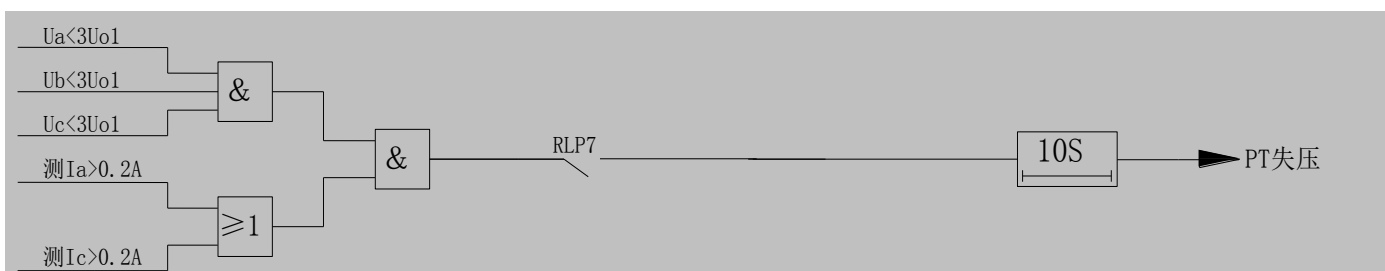
图 5 PT 失压报警逻辑框图
