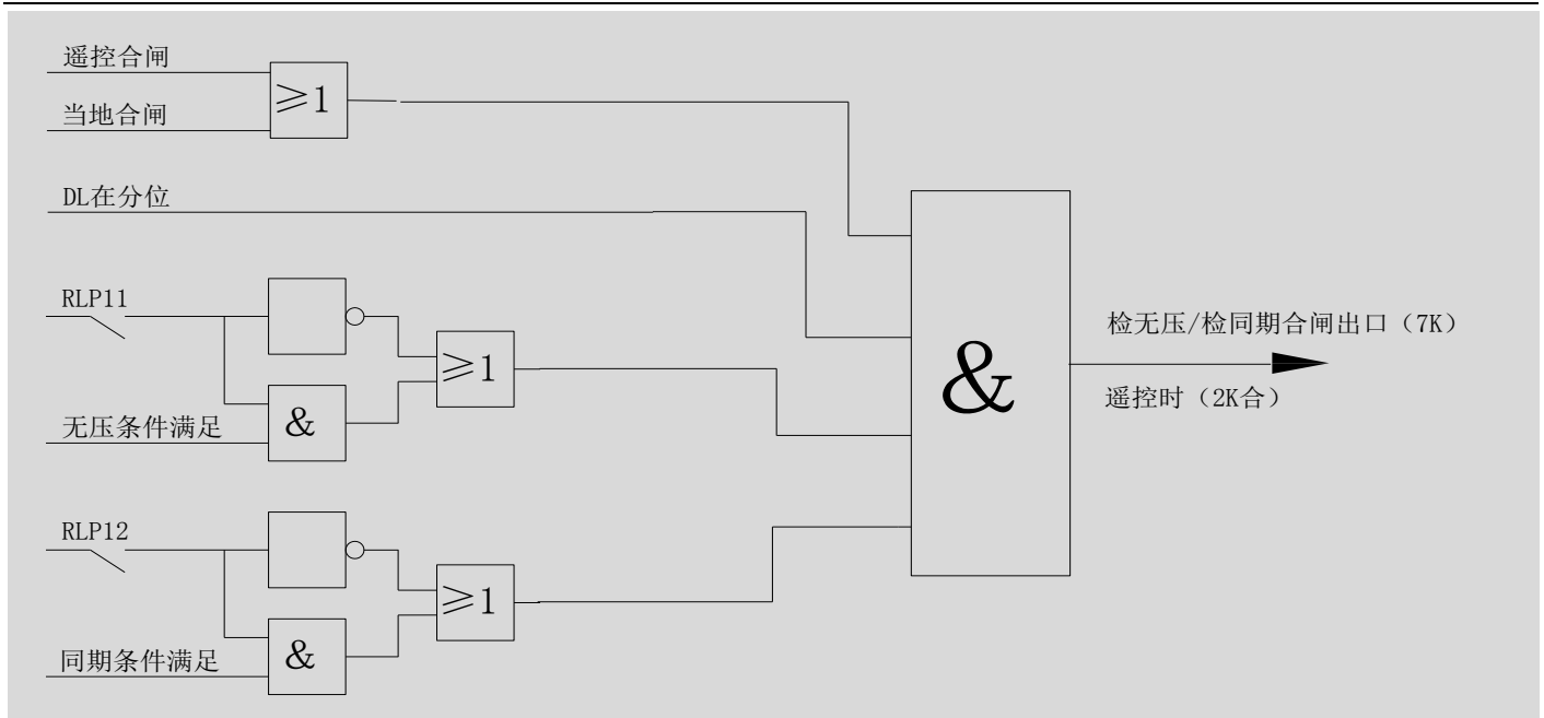
图 7 检同期/检无压合闸逻辑框图
