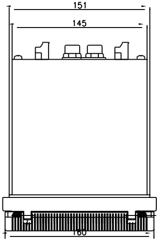
SDP-3000系列保护测控装置顶视图
