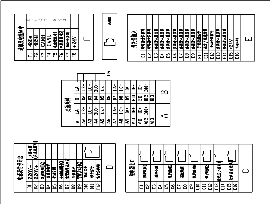
SDP-3024 变压器低后备保护测控装置背板端子图
