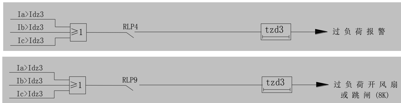
图 2 过负荷保护逻辑框图
