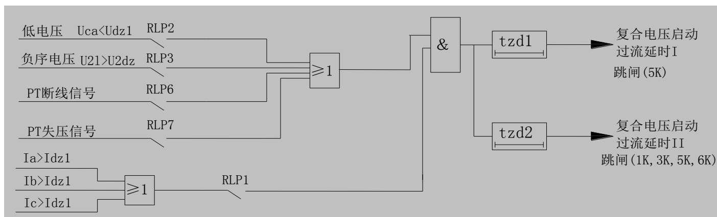
图 1 过流保护逻辑框图
