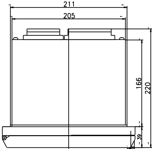
SDP-3000系列保护测控装置侧面图
