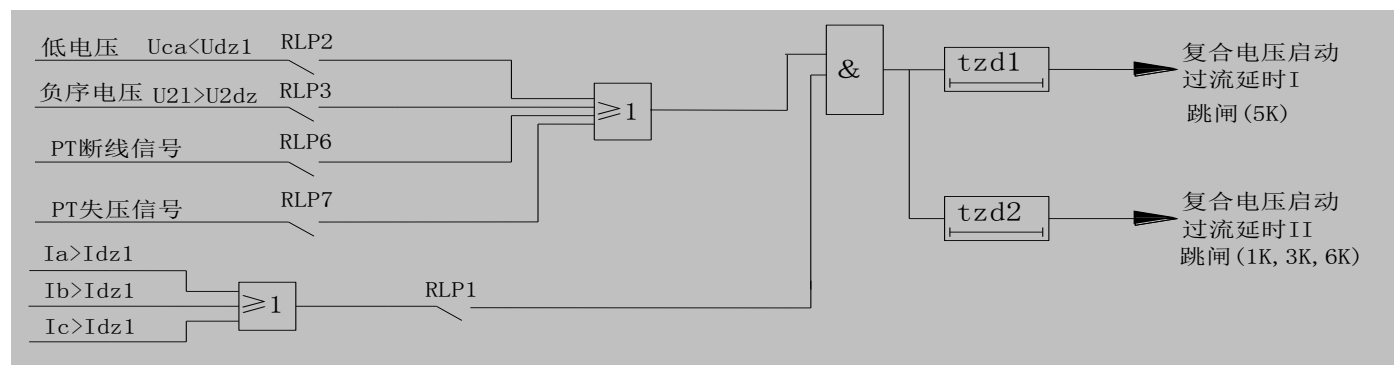
图 1 过流保护逻辑框图
