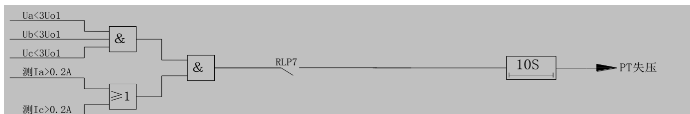
图 5 PT 失压报警逻辑框图
