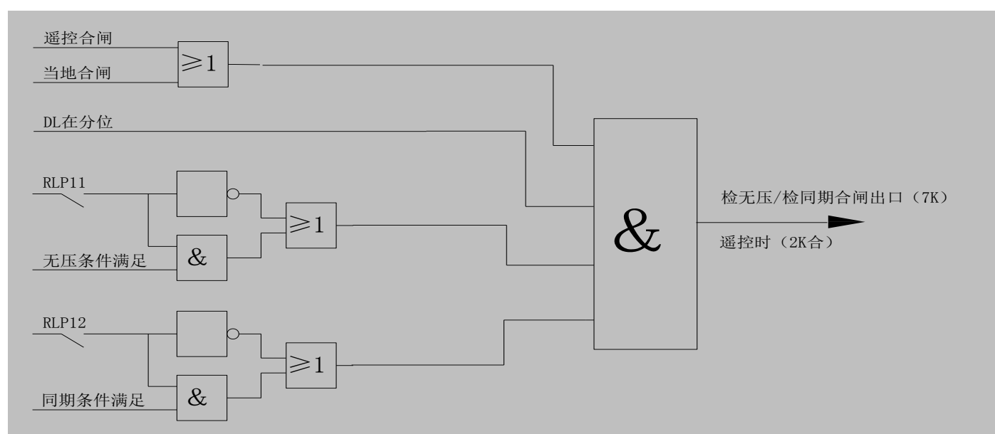
图 7 检同期/检无压合闸逻辑框图
