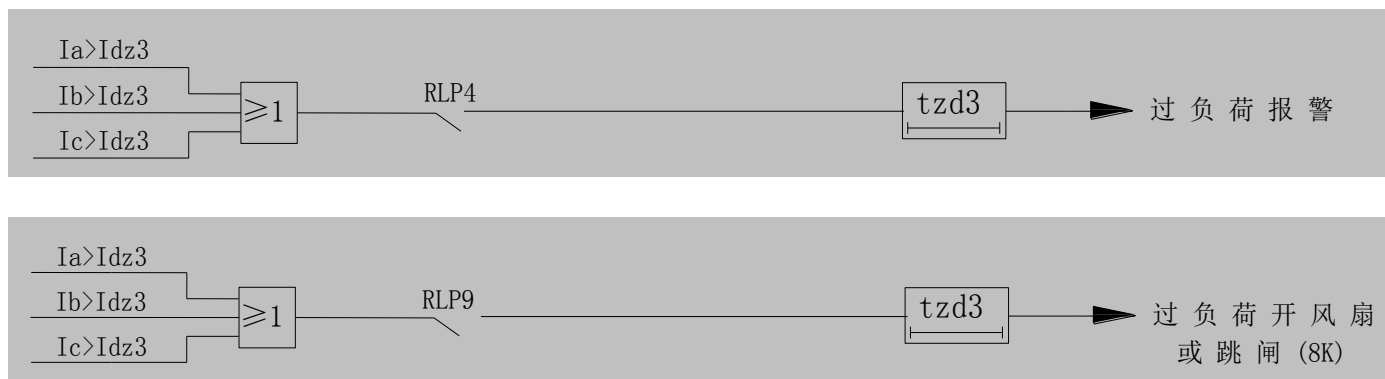
图 2 过负荷保护逻辑框图
