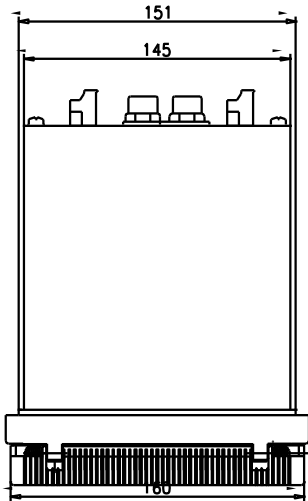
SDP-3000系列保护测控装置顶视图
