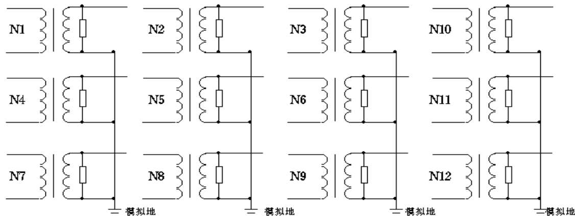
交流采样模件原理图
