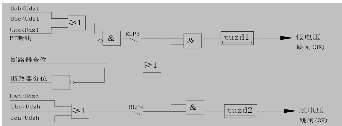
图 2 低电压、过电压保护逻辑图
