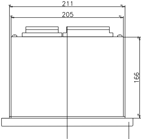
SDP-3000 系列保护测控装置侧面图
