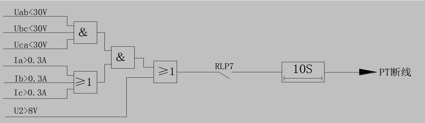
图 4 PT 断线逻辑图
