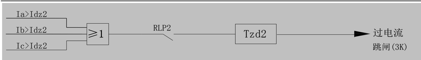
图 1 二段电流保护逻辑图
