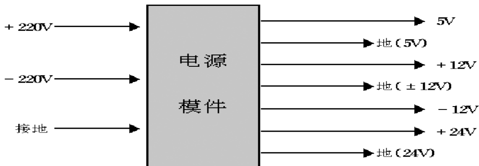
电源模件示意图
