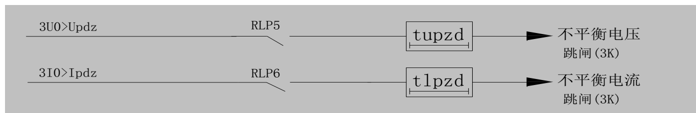
图 3 不平衡电压（电流）逻辑图
