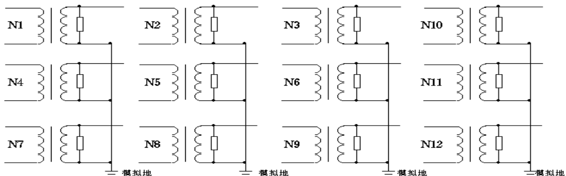
交流采样模件原理图
