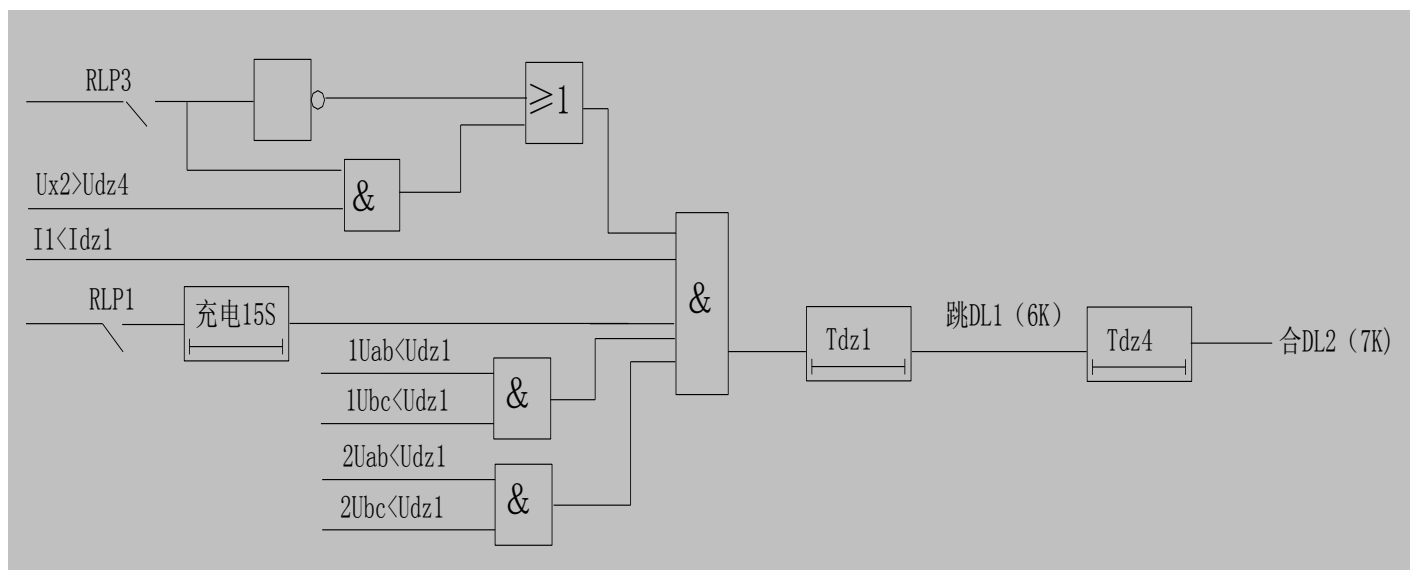
图 2 自投方式 1 逻辑图
