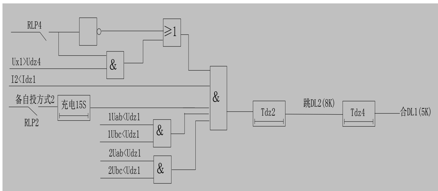
图 3 自投方式 2 的逻辑图
