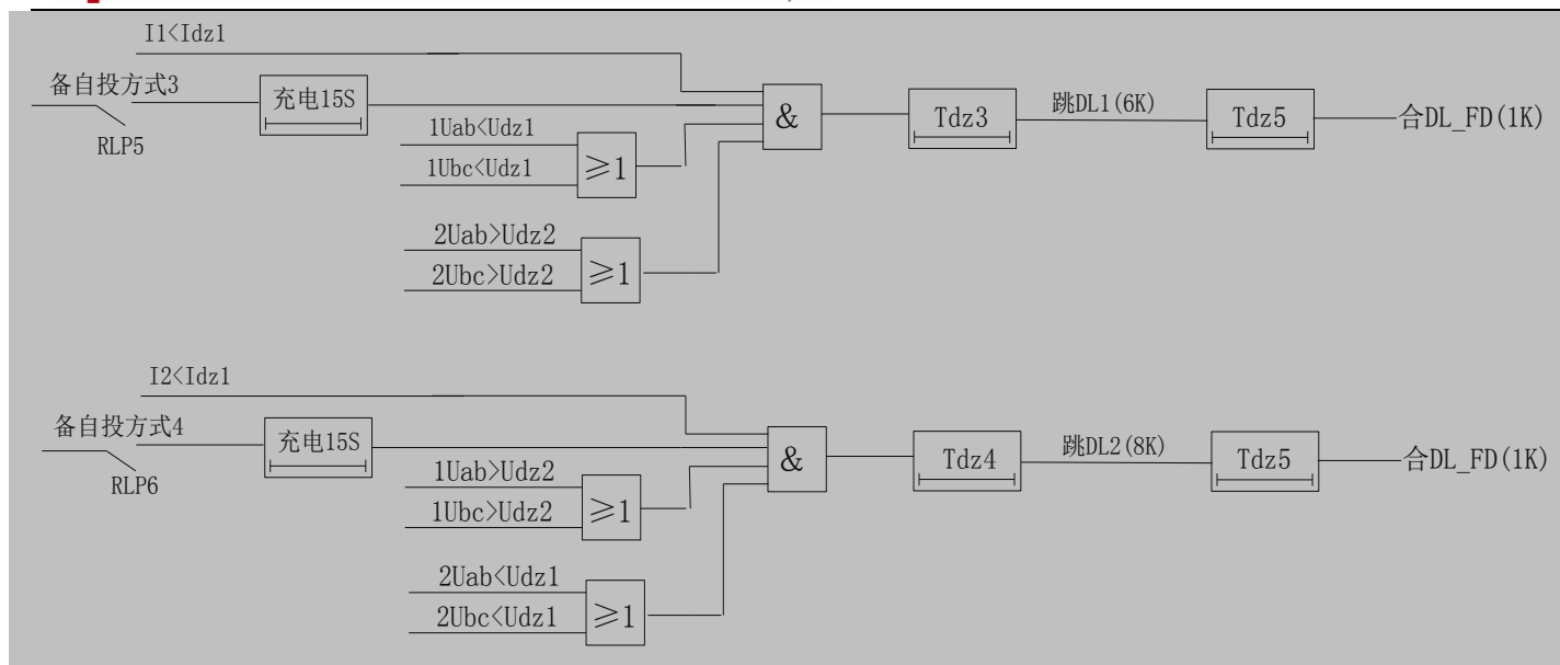
图 4 自投方式 3、4 的逻辑图
