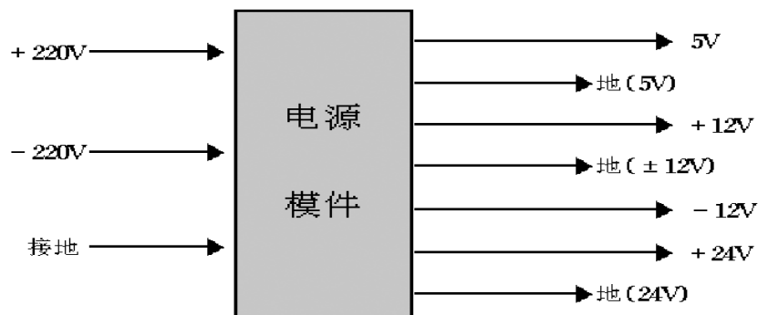
电源模件示意图
