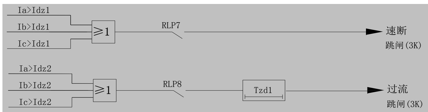
图 5 两段式保护逻辑图
