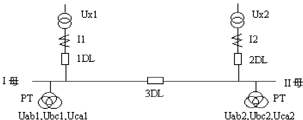
图 1 系统主接线
