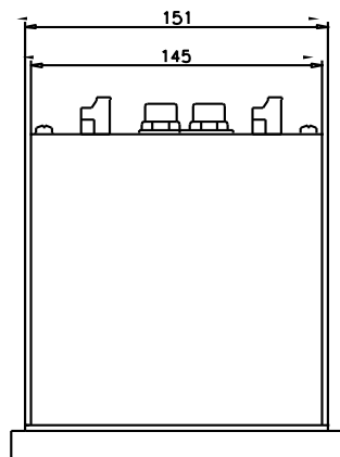
SDP-3000系列保护测控装置顶视图
